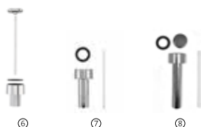
Conjunto pulsador elevado (tapa Ø27)
